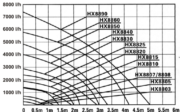
VÝKONNOSTNÍ KŘIVKA
