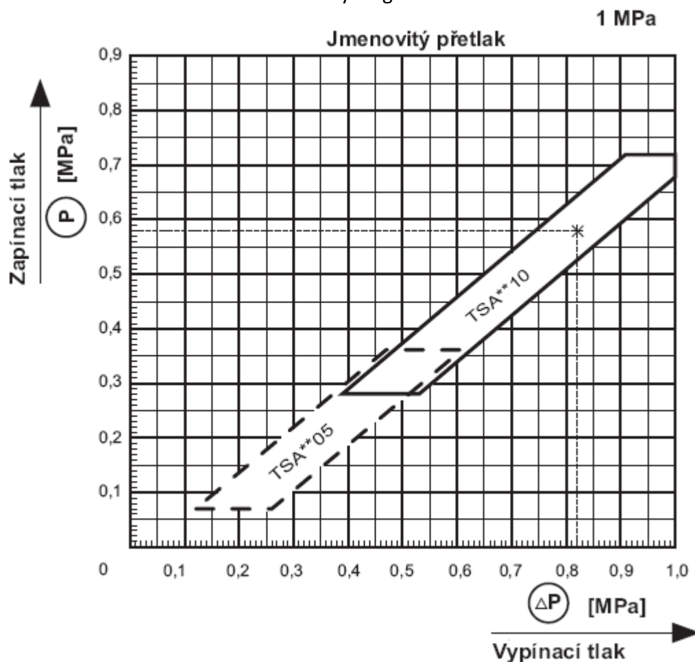
Tlakový diagram
